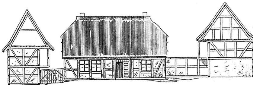
Ryc. 10. Przekrój tradycyjnej zagrody pomorskiej (źródło: Das Bauernus 1990)
